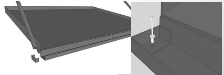
Rännin vedenohjauksen toisen pään sulkeminen
